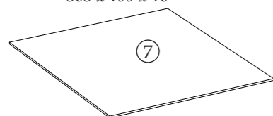
Trasera / Back panel / Arrière / Traseira 434 x 376 x 3
