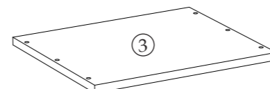
Tapa / Top / Toit / Tampa 402 x 340 x 16
