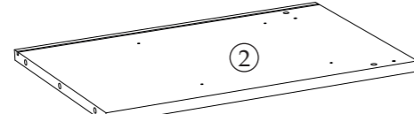
Costado izquierdo / Left side / Côté gauche / Lado esquerdo 484 x 338 x 16
