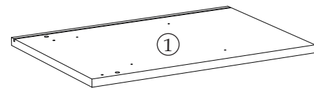
Costado derecho / Right side / Côté droit / Lado direito 484 x 338 x 16
