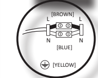
4 Realizamos la conexión a la ficha que se adjunta.
