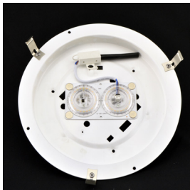
5 Se instala en la base de la luminaria mediante imanes incorporados en la placa.
