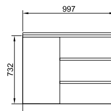
Ancho 1005 3 cajones + 1 puerta
